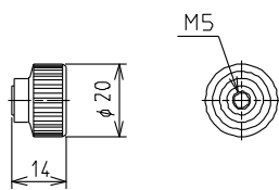
(3) Knob
